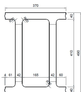
tvárnice krajová
