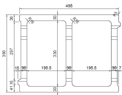
tvárnice průběžná
