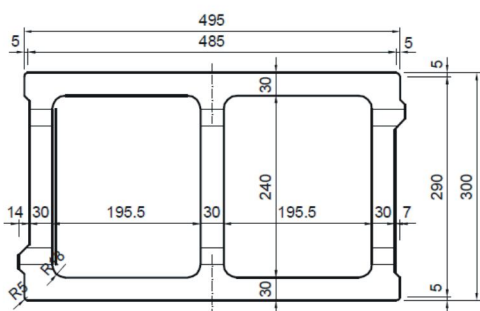
tvárnice průběžná
